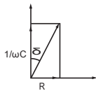
图10：损失角 \tan\delta
