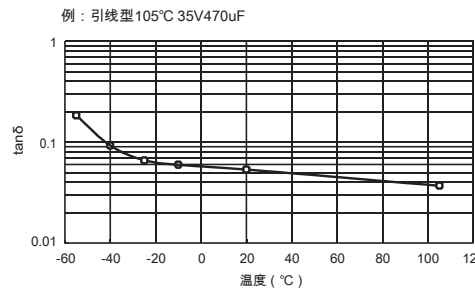
图11： \tan\delta 的温度特性
