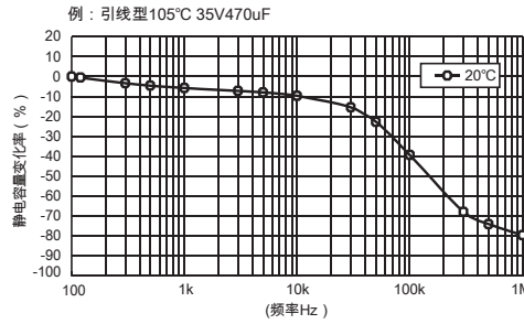
图8：静电容量的频率特性
