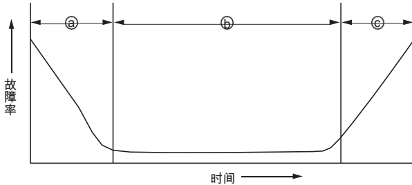
图17：浴桶曲线
