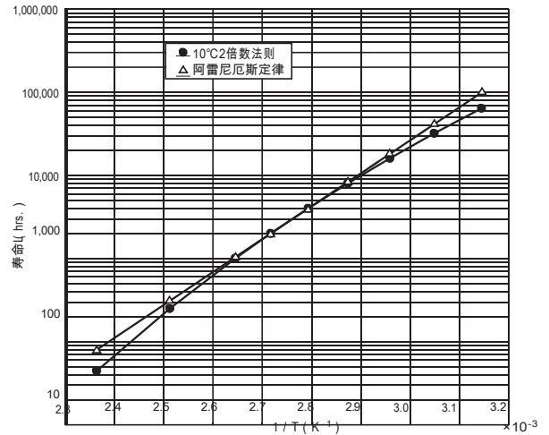
图19：阿雷尼厄斯定律和10°C2倍数的寿命计算结果
