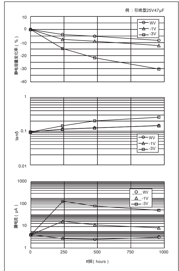
图27：105°C反相电压特性
