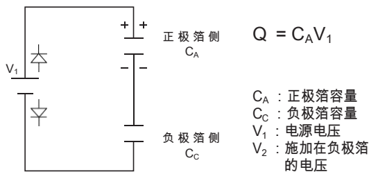
图21：充电时的电荷状态
