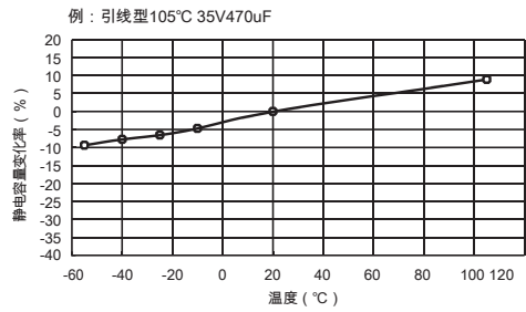
图7：静电容量的温度特性
