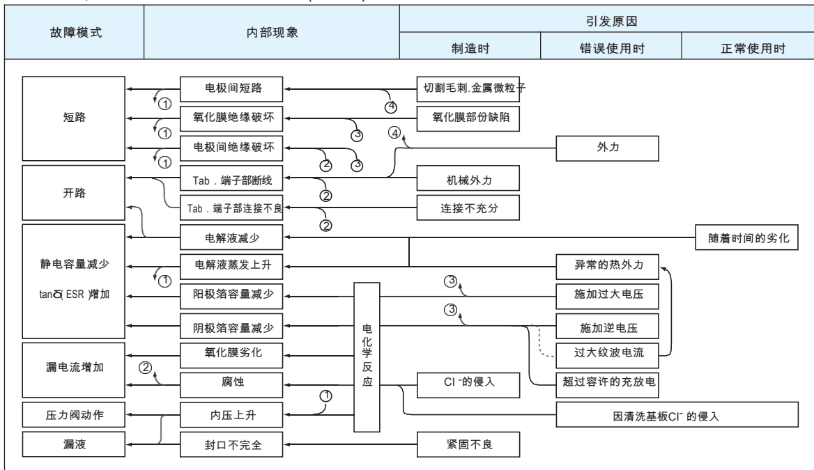
图18：故障模式
